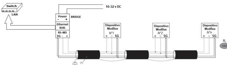
→ Fig.6 Schema di collegamento
