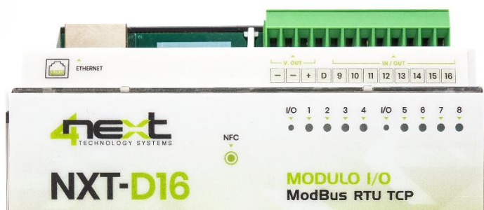
Fig. 3/a Parte superiore
