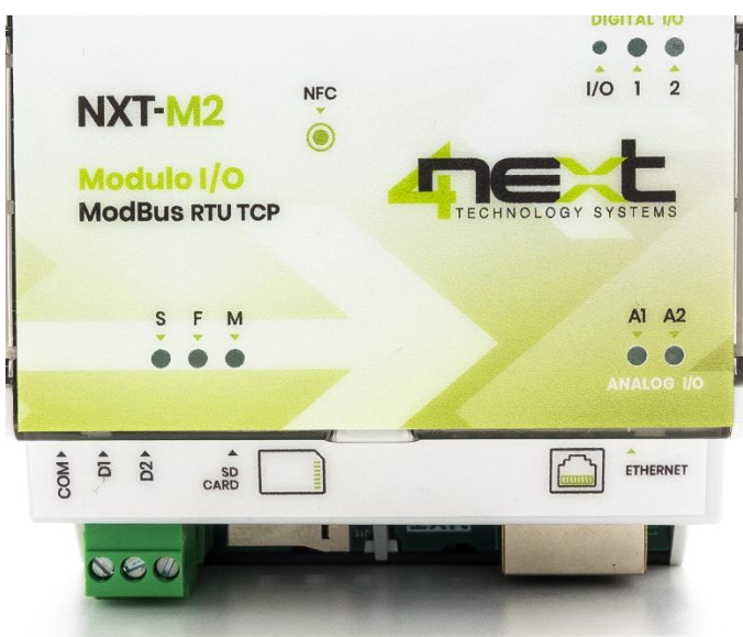
Fig. 3/c Parte inferiore
